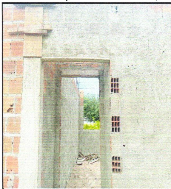
FOTO- 20 CONTRAVERGA MOLDADA IN LOCO COM UTILIZAÇÃO DE BLOCOSCANALETA,
