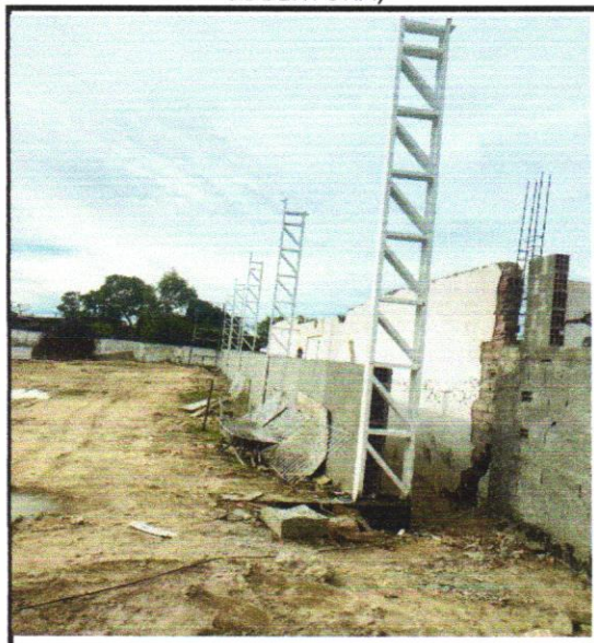
FOTO - 03 : ESTRUTURA TRELIÇADA DE COBERTURA;
