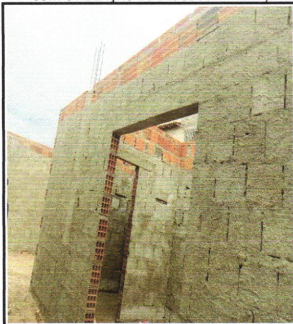
FOTO - 18 CONTRAVERGA MOLDADA IN LOCO COM UTILIZAÇÃO DE BLOCOSCANALETA,
