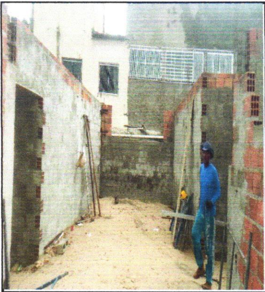
FOTO 11-ALVENARIA DE VEDAÇÃO DE BLOCOS CERÂMICOS FURADOS NA HORIZONTAL DE 9X19X19 CM (ESPESSURA 9 CM) E
