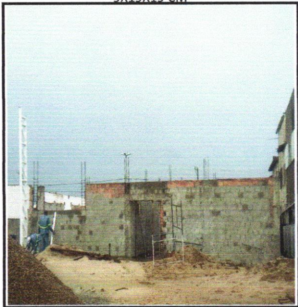
FOTO - 10 ALVENARIA DE VEDAÇÃO DE BLOCOS CERÂMICOS FURADOS NA HORIZONTAL DE 9X19X19 CM
