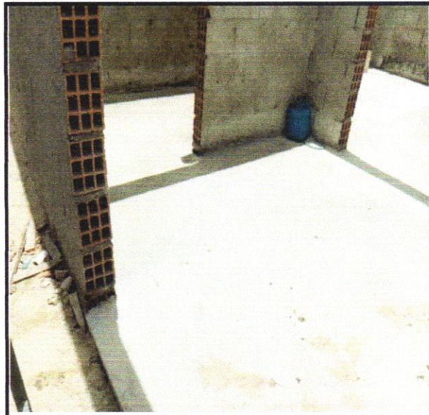
FOTO - 08 LASTRO DE CONCRETO MAGRO, APLICADO EM PISOS, LAJES SOBRE SOLO OU
