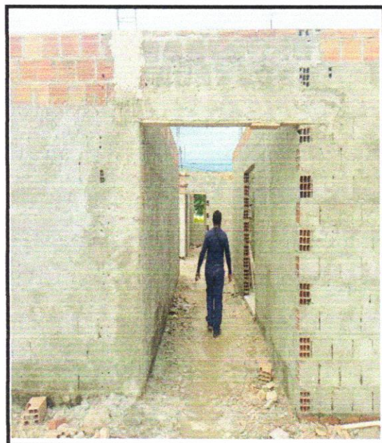
FOTO 19- CONTRAVERGA MOLDADA IN LOCO COM UTILIZAÇÃO DE BLOCOSCANALETA, ESPESSURA DE *20* CM. AF_03/2024
