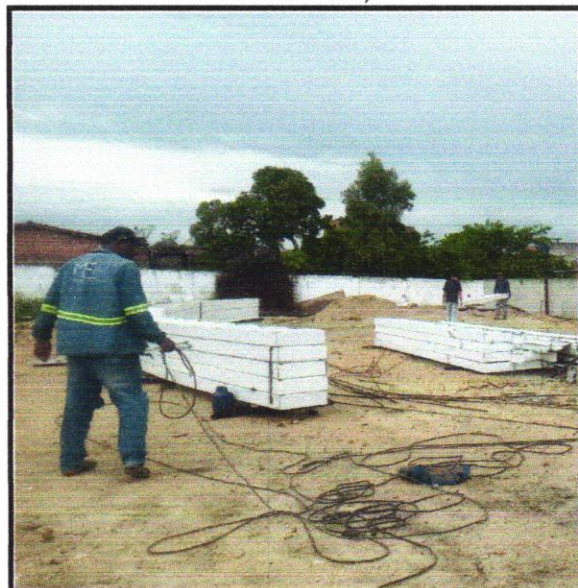
FOTO - 04: ESTRUTURA TRELIÇADA DE COBERTURA;
